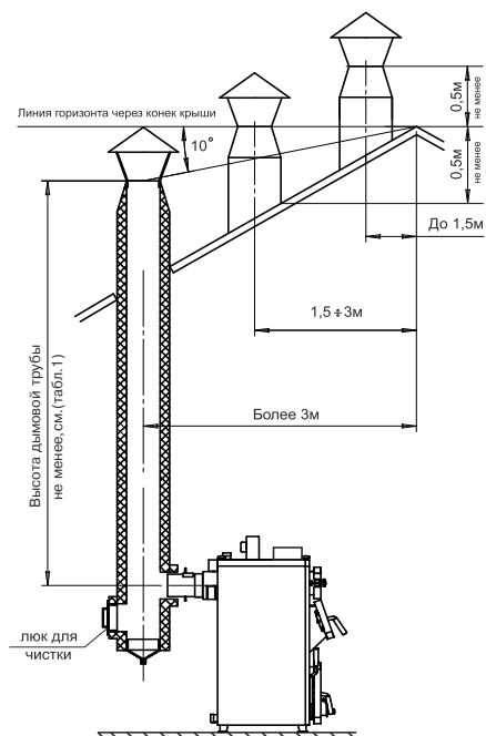
Рис.6 Варианты установки дымоходной трубы
